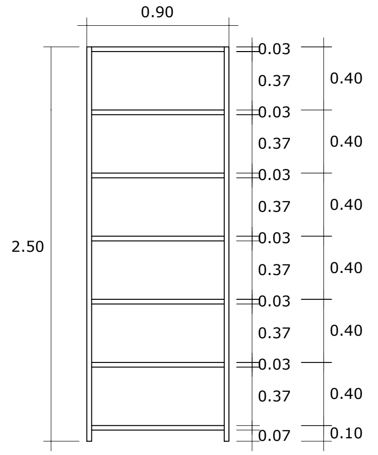
CORTE 3 - 3' ESC: 1/25
