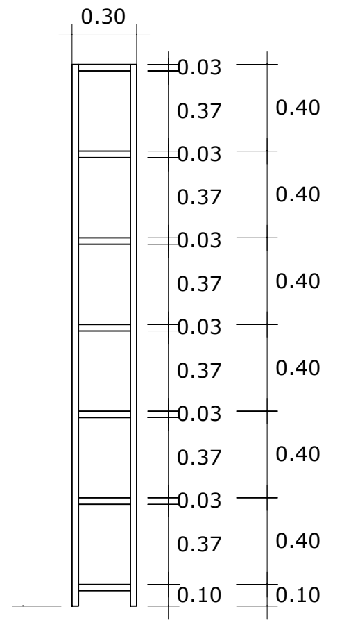
CORTE 4 - 4' ESC: 1/25
