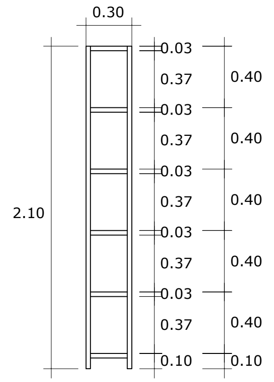
CORTE 2 - 2' ESC: 1/25
