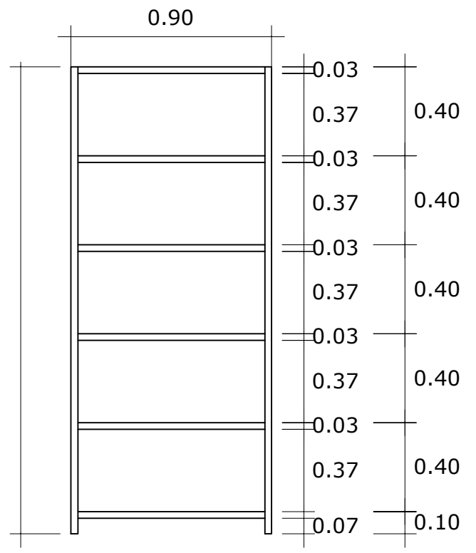
CORTE 1 - 1' ESC: 1/25
